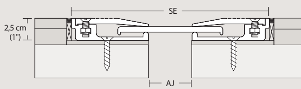
AL-HD Modelo AL-HD específico para servicio pesado. Para cargas móviles de 907,18 kg (2000 lb).
