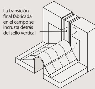
Transiciones de parapeto
