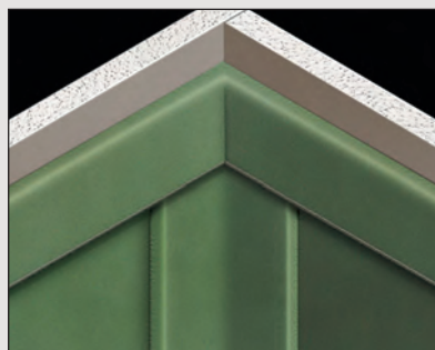
Esquina interior de altura parcial (10mm o 3/8" de grosor) Incluye guarnición horizontal de 13mm (1/2") de grosor
