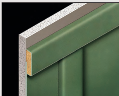
Moldura de friso (wainscot) estándar (13mm o 1/2" de grosor) También disponible en opción de guarnición colonial*
