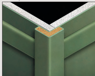
Esquina exterior de altura completa (16mm o 5/8" de grosor) Incluye guarnición horizontal de 13mm (1/2") de grosor
